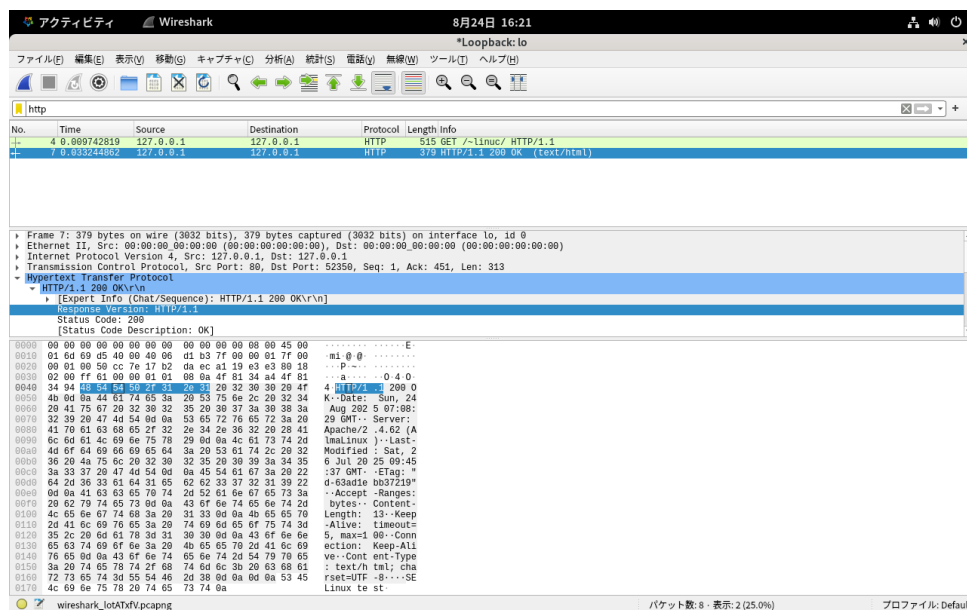
図 17: http で絞り込みを行います
