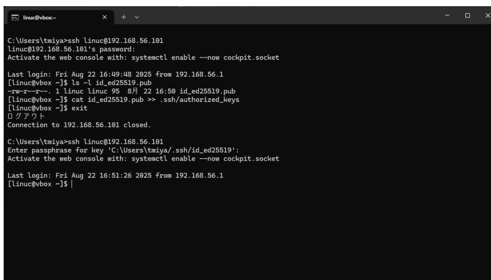
図 12: 公開鍵認証で Linux にリモートログイン
