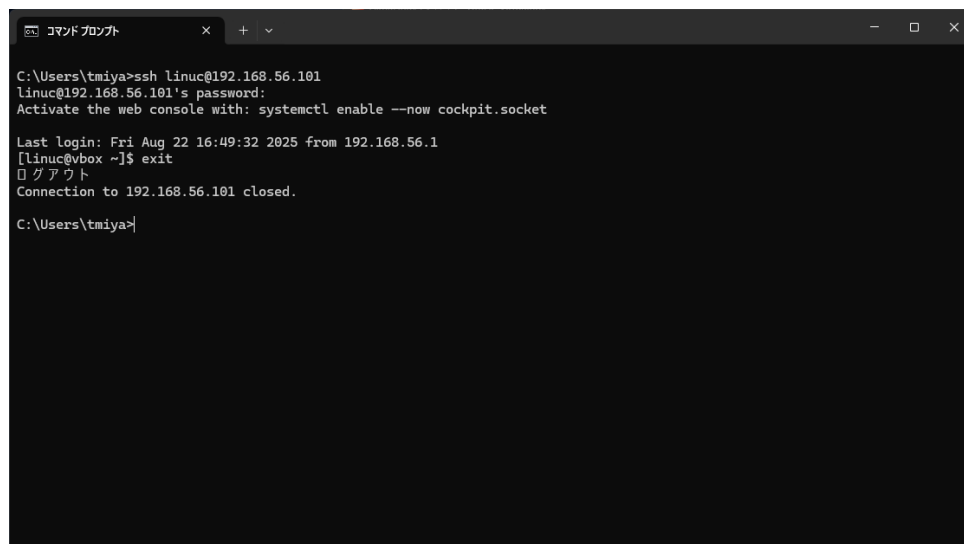
図 9: パスワード認証で Linux にリモートログイン
