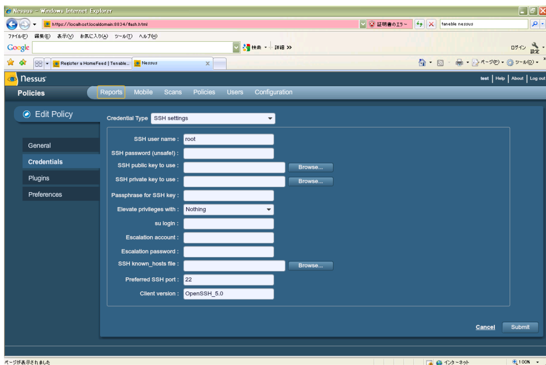
図 8.19 Nessus の管理画面（ポリシー編集画面）
