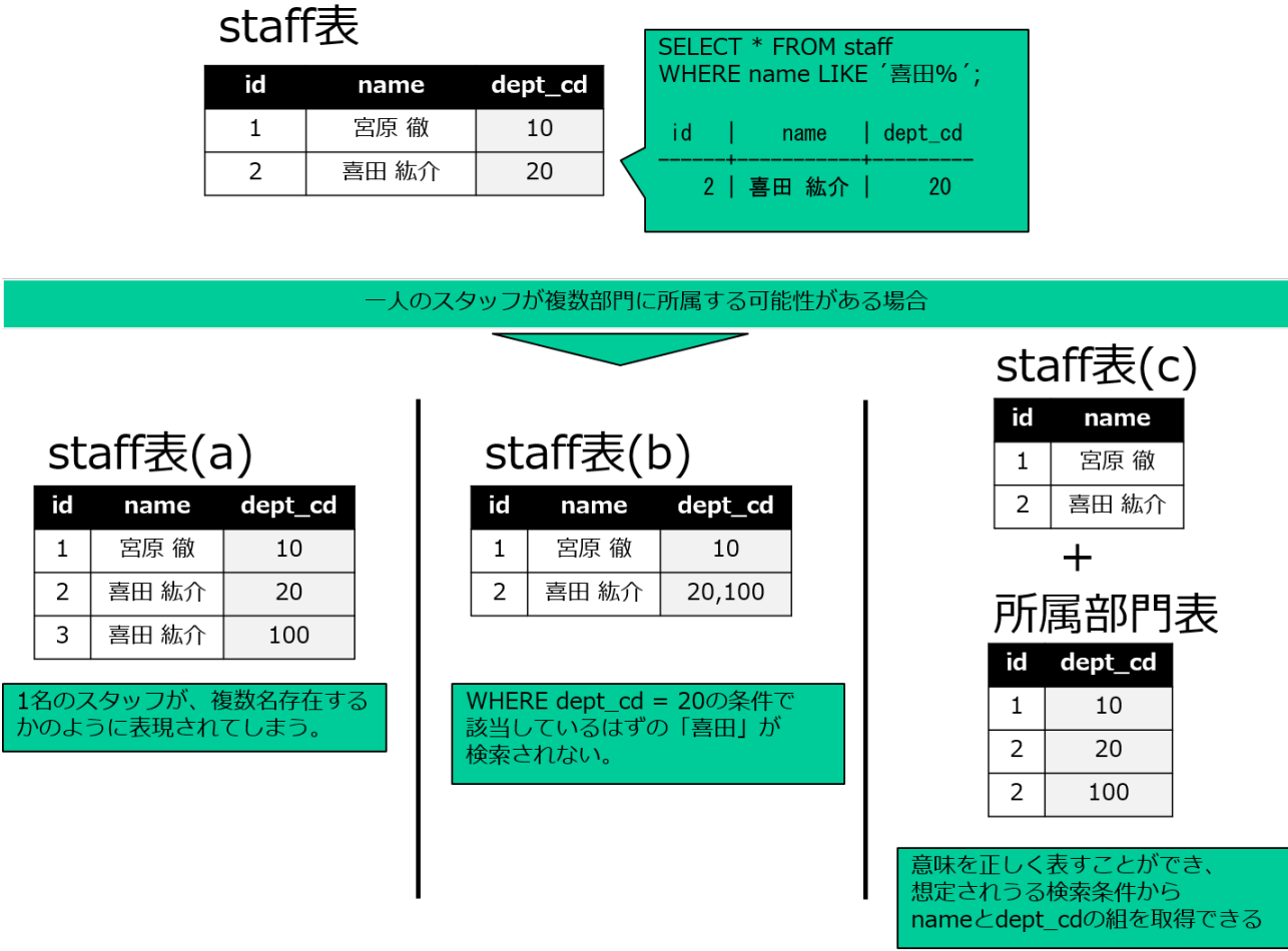
図 8: ALTER TABLE は行うべきか
