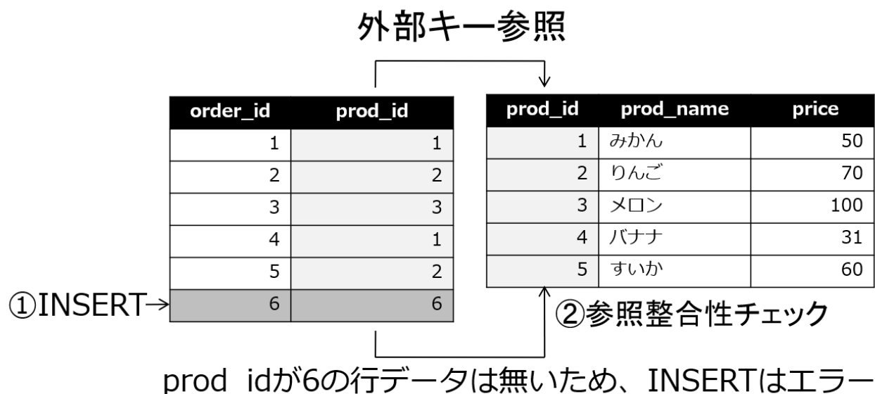
図 9: 外部キー制約違反
